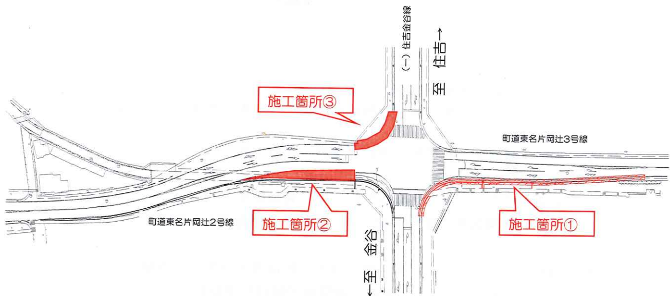
計画工程表
